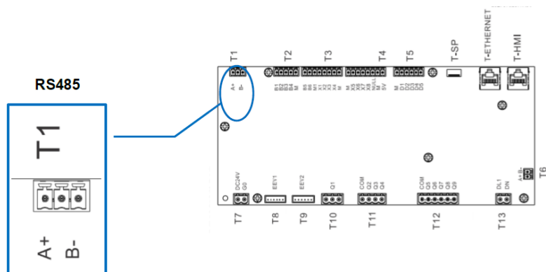
Figura 11 - Puerto Modbus de la unidad Daikin
