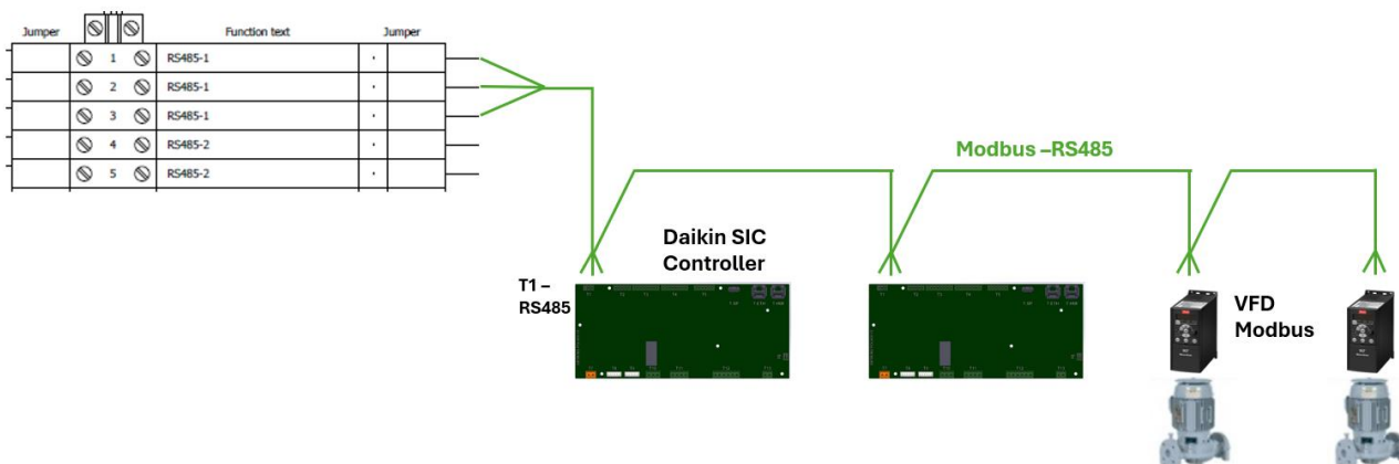
Figura 9 - Red de equipos del lado de agua
