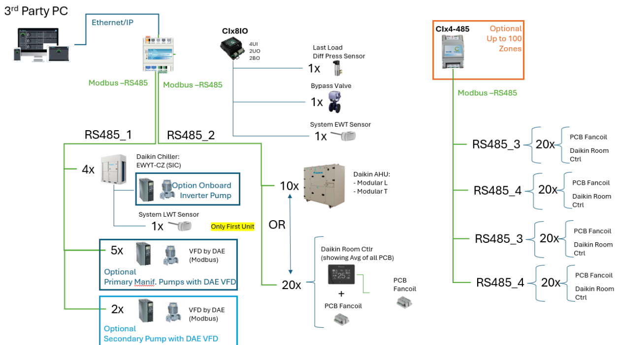
Figura 7 - Arquitectura de cables y redes
