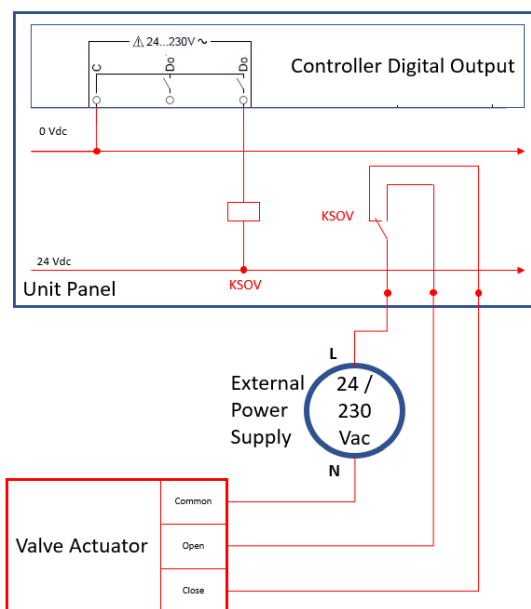
Figura 6 - Instalación eléctrica de la válvula de cierre
