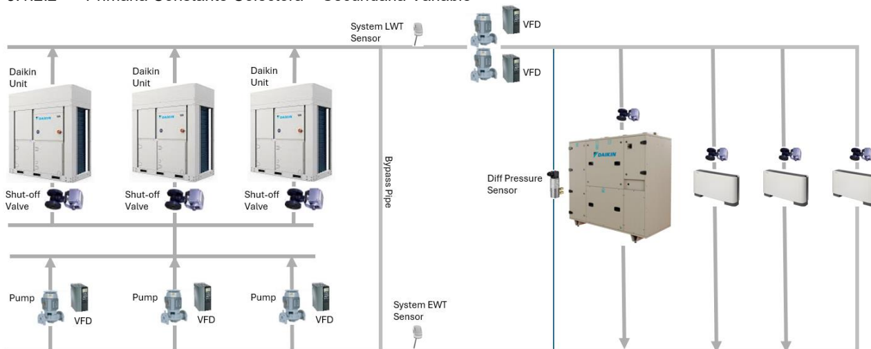
Figura 5 - Primaria Constante Colectora – Secundaria Variable
