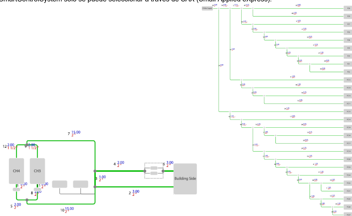
Figura 1 - Planta de agua SAX y diseño del lado aire
