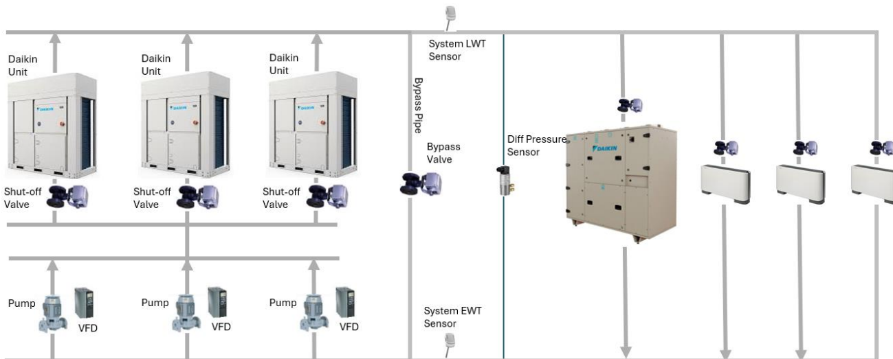
Figura 3 - Sólo variable primaria con colector
