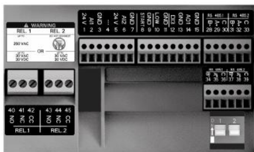
Figura 13 - Placa de terminales HydrovarX EXM
