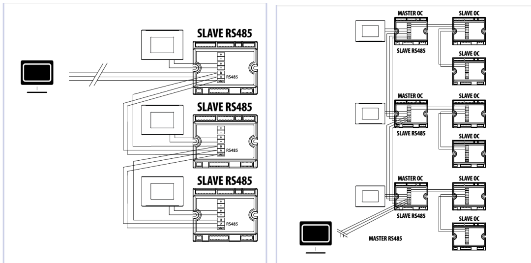
Figura 12 - FWTOUCH - Configuración de la red Modbus
