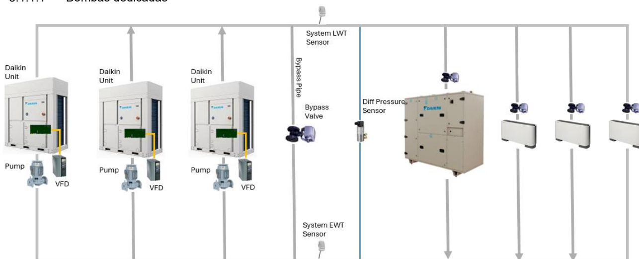
Figura 2 - Sólo variable primaria dedicada
