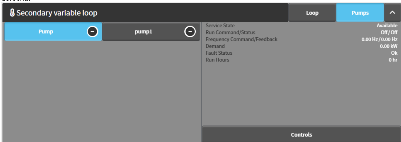
Figura 73 – Widget de bomba - Datos
