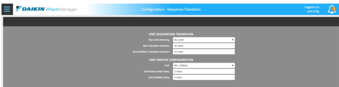
Figura 37 - Configuración de transición de secuencia
