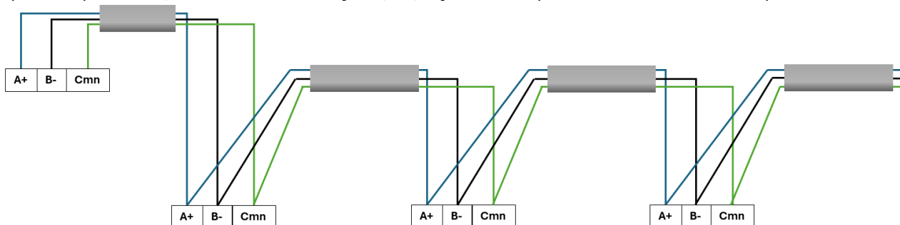
Figura 8 - Ejemplo general de red Modbus
