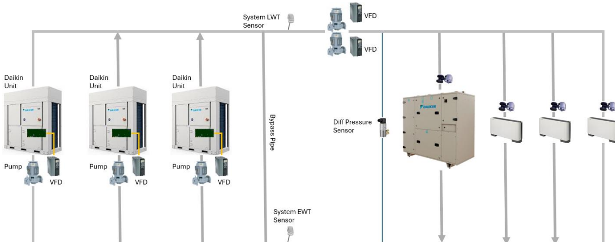
Figura 4 - Primaria Constante Dedicada – Secundaria Variable
