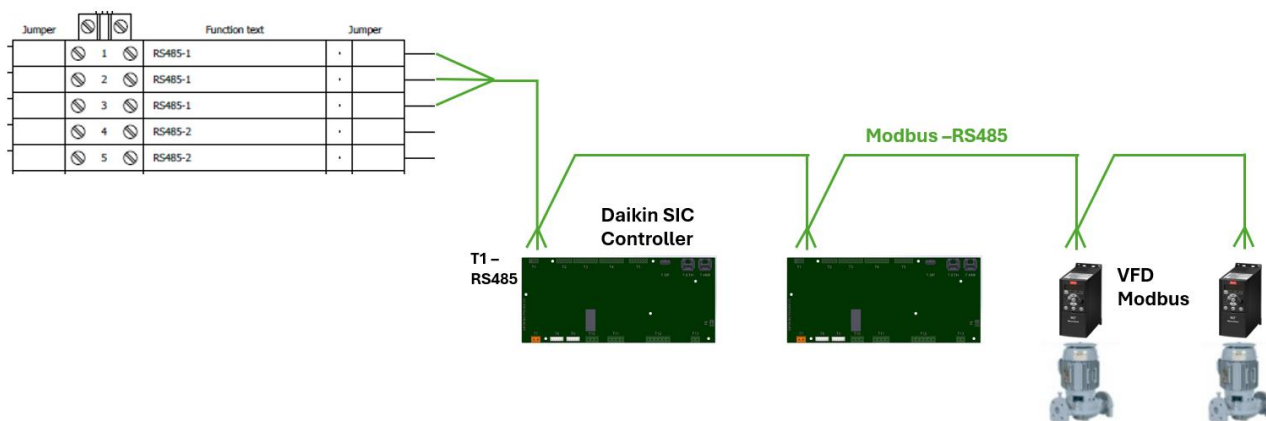
Figure 9 - Réseau équipement côté eau
