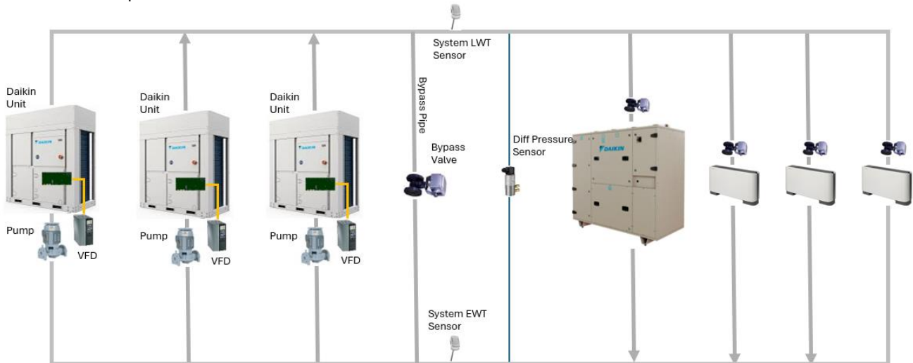
Figure 2 - Variable primaire dédiée uniquement
