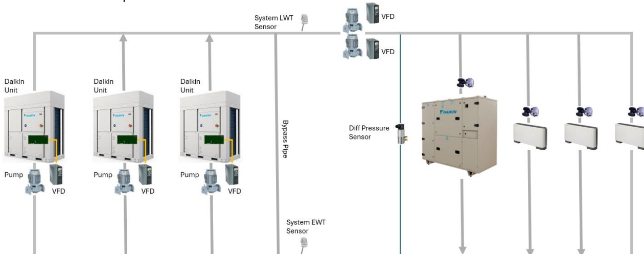
Figure 4 - Constante primaire dédiée - Variable secondaire
