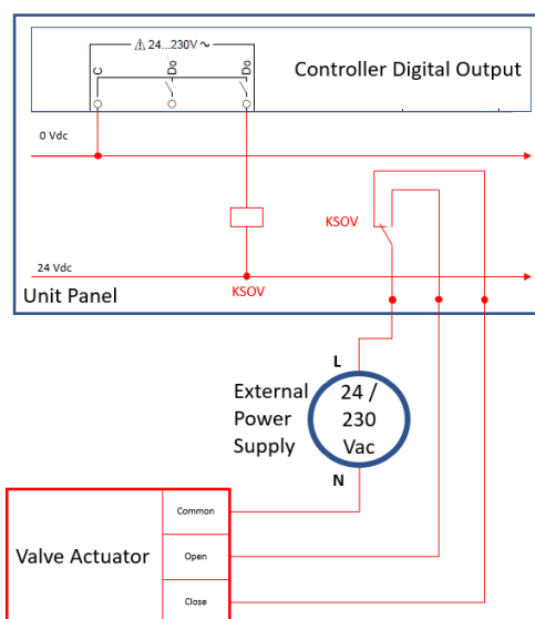
Figure 6 - Installation électrique de la vanne d'arrêt
