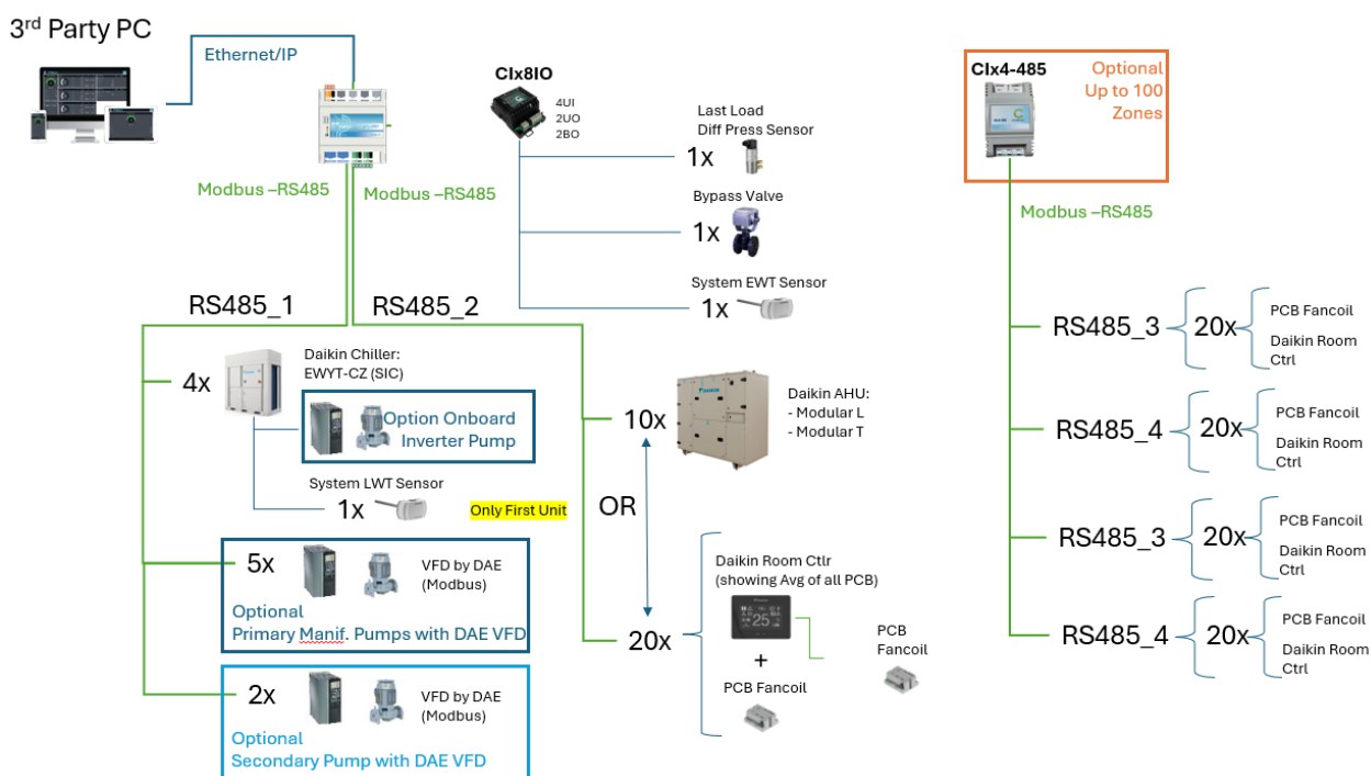
Figure 7 - Architecture du câble et du réseau
