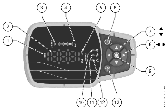
Figure 14 - Écran HydrovarX
