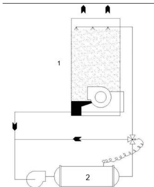
Fig.° 7- Schéma de contrôle du condenseur avec tour de refroidissement
