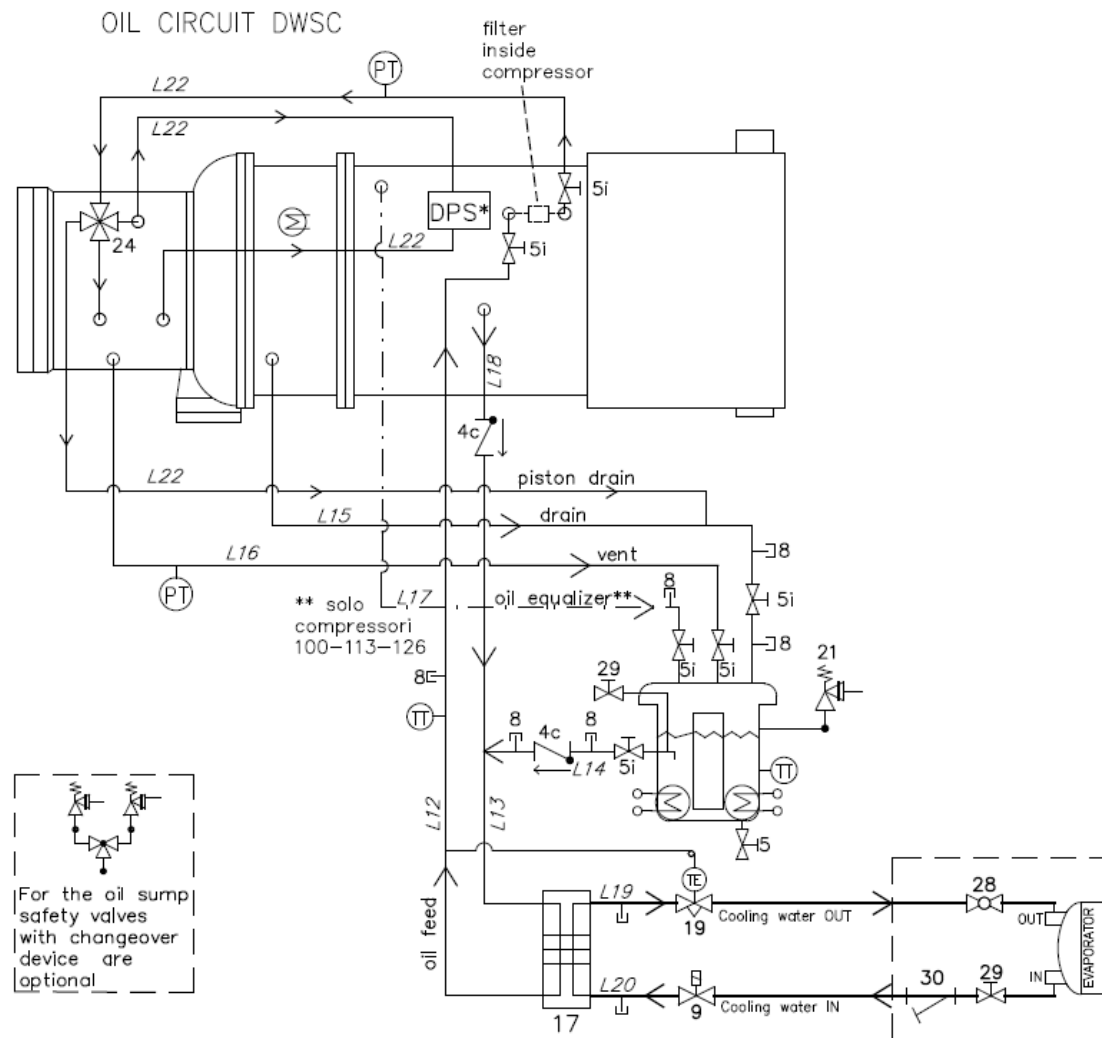
Fig.° 2 - Circuit d'huile type
