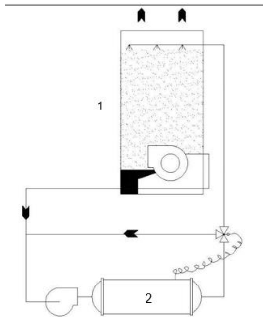
Obr. 7 – Systém řízení kondenzátoru s chladicí věží
