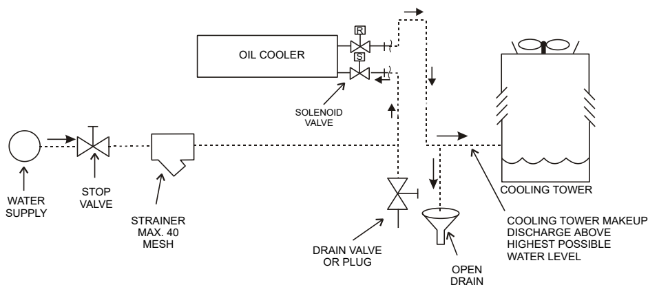
Fig. 10 - Enfriador de aceite refrigerado con agua de la red pública
