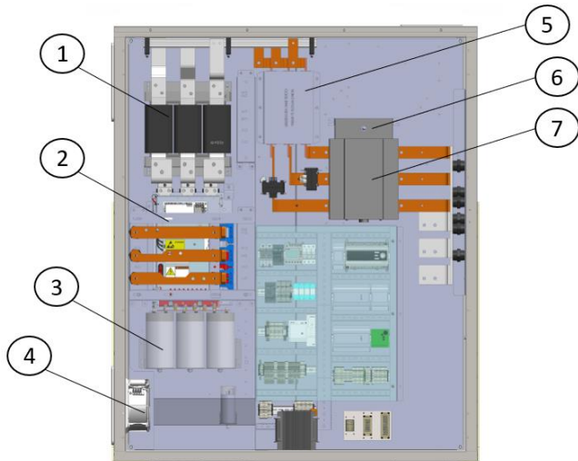
Fig. 24 - Elementos del panel inverter (doble)
