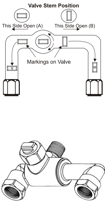
Fig.º 13 - Dispositivo de cambio
