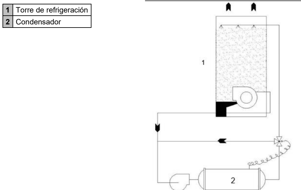
Fig. 7 - Esquema para el control de la condensación con torre de evaporación
