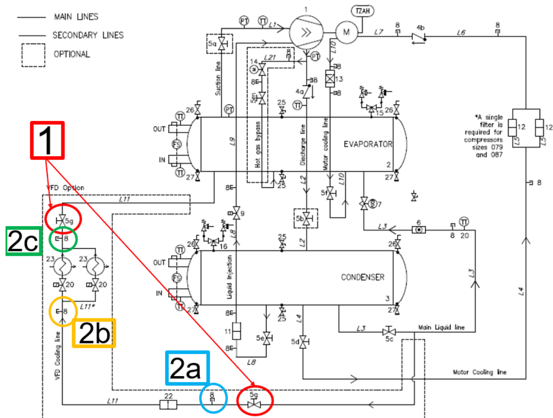
Fig.° 30 - Schéma P&ID de l'unité avec détail de la ligne de refroidissement de l'onduleur
