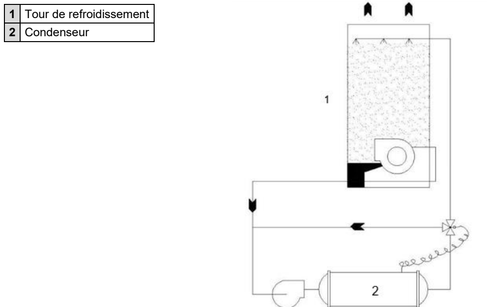
Fig.° 7- Schéma de contrôle du condensateur avec tour de refroidissement
