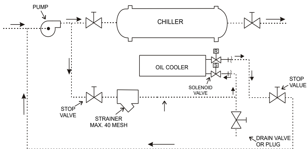
Fig.° 9- Tubazioni del raffreddatore dell'olio attraverso la pompa dell'acqua refrigerata
