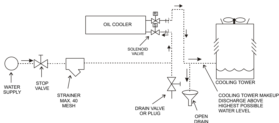
Fig.° 11- DWSC, collegamenti di raffreddamento dell'olio
