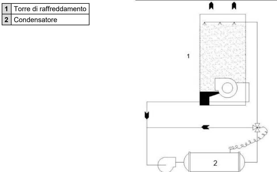
Fig.° 7- Schema di controllo del condensatore con torre di raffreddamento
