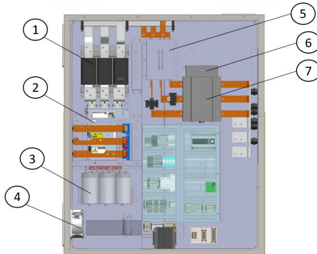
Fig.° 24- Parti del pannello inverter (doppio)
