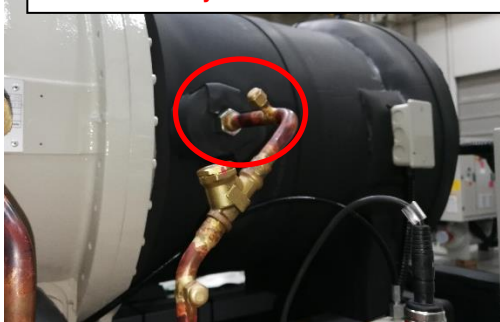
Motorház nyomáscsökkentő kiemenet
