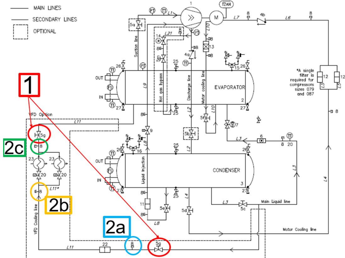
25. ábra - A berendezés P&ID rajza az inverter hűtési vezetékek részleteivel
