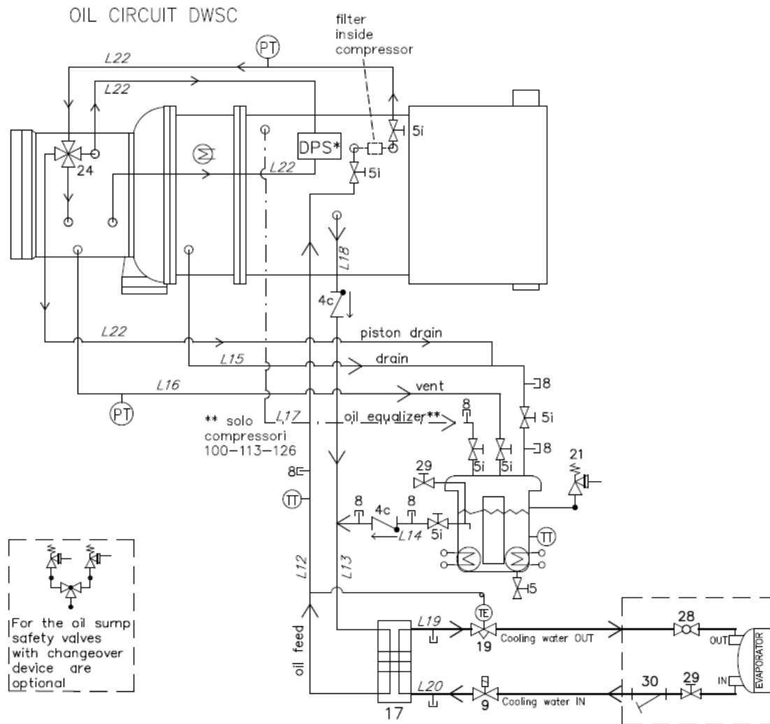
Afb. 2 - Voorbeeld oliecircuït
