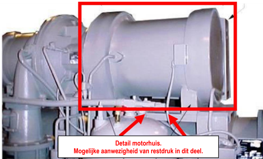
Drukpoort motorhuis
