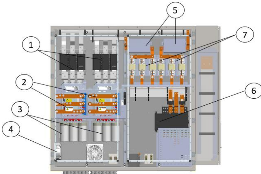
Obr. 26 - Součásti panelu měniče (duální)
