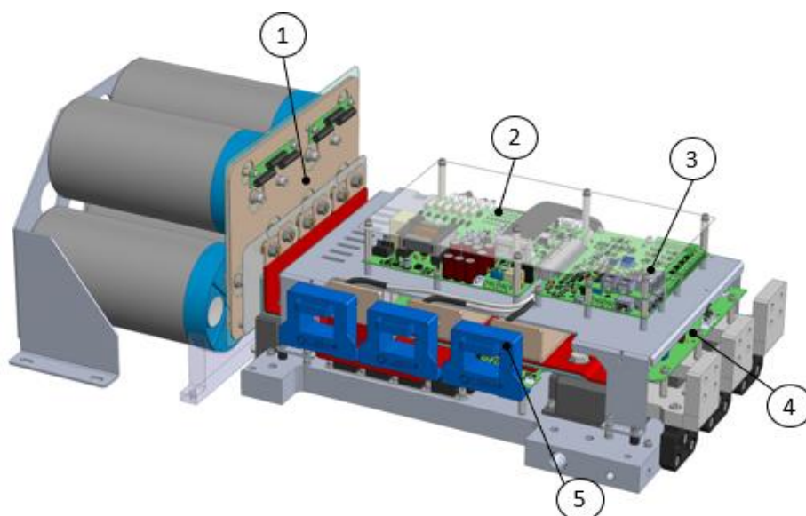
Obr. 27 - Označení vyměnitelných částí VFD
