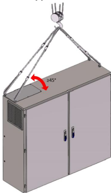
Obr. 17 - Úhel, který je nutno dodržovat při zvedání
