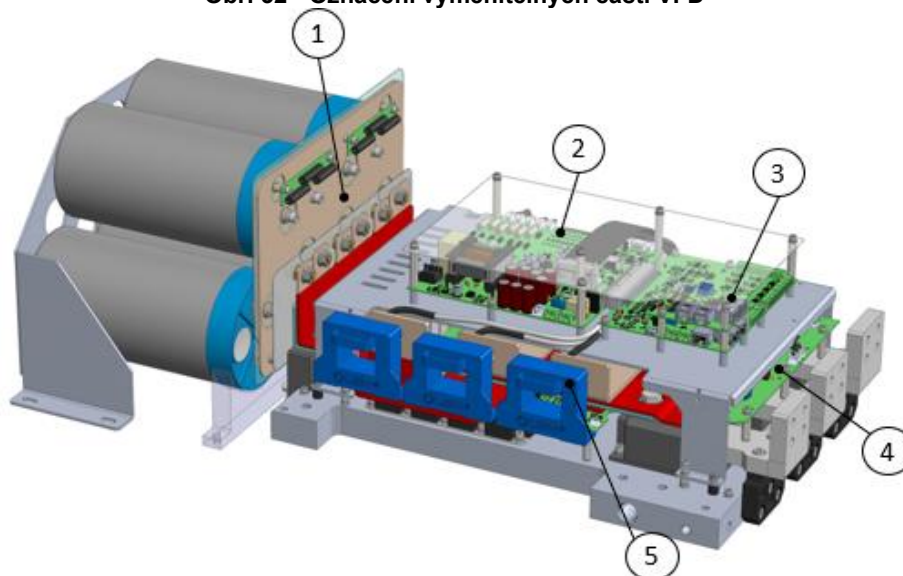
Obr. 32 - Označení vyměnitelných částí VFD
