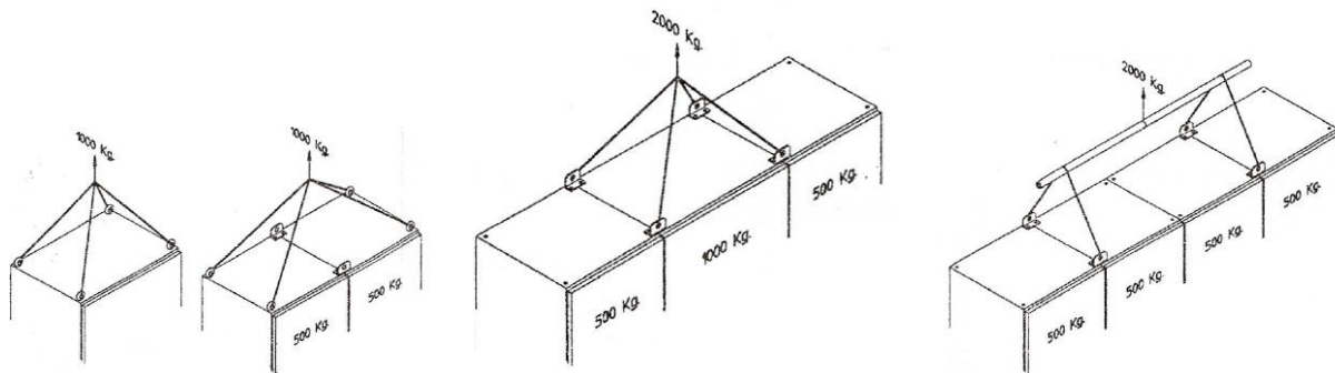
Obr. 18 - Zvedání VFD
