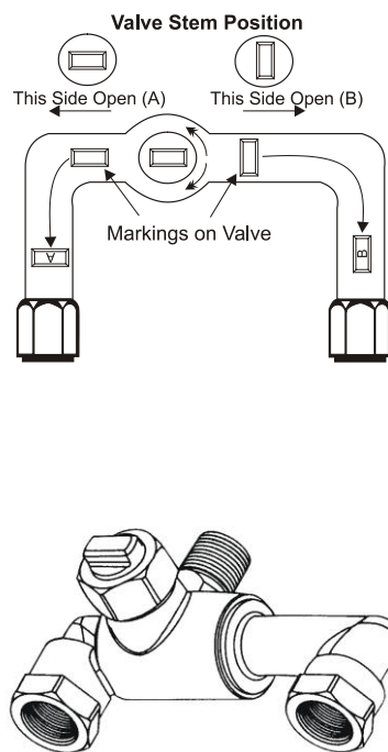
Obr.°13 - Přepínací zařízení
