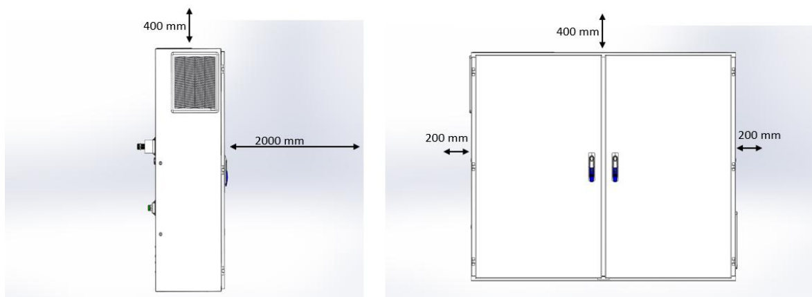
Obr. 19 - Minimální prostorové požadavky pro VFD
