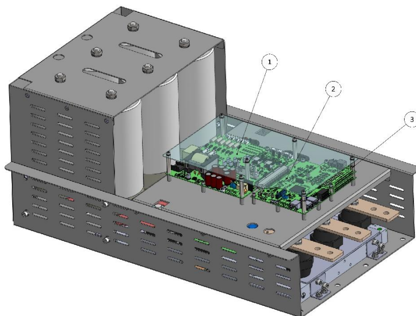
Obr. 33 - Označení vyměnitelných částí aktivního filtru
