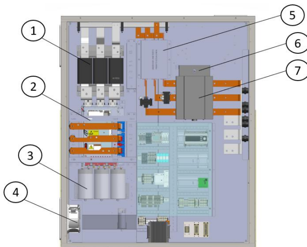
Obr. 26 - Součásti panelu měniče (duální)
