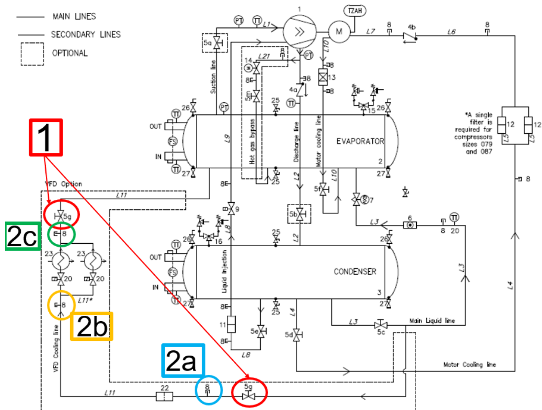
Obr. 28 - Diagram P&ID jednotky s detailem chlazení měniče
