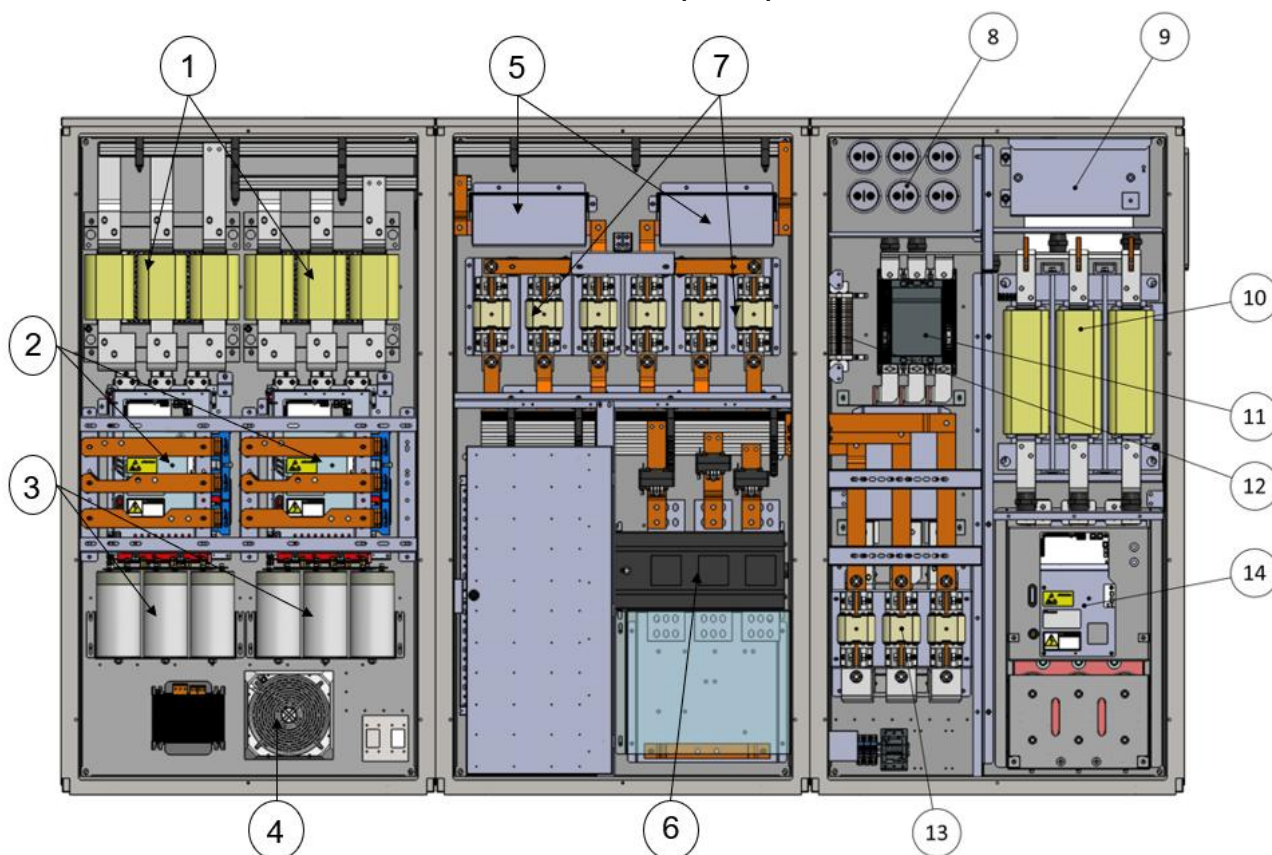
Obr. 31 – VFD se součástmi panelu pro aktivní filtr
