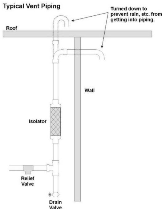
Obr.°12 - Typické odvězdušňovací potrubí
