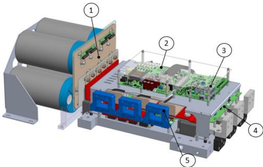
Abb.° 26 - Austauschbare Teile des VFD hervorgehoben
