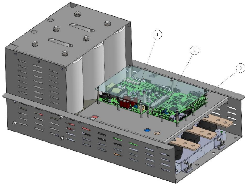
Abb.° 32 - Austauschbare Teile des aktiven Filters hervorgehoben
