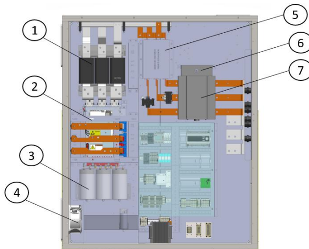
Abb.° 25 - Teile der Inverter-Schalttafel (Dual)
