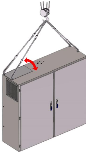
Abb.° 16 - Beim Heben einzuhaltender Winkel
