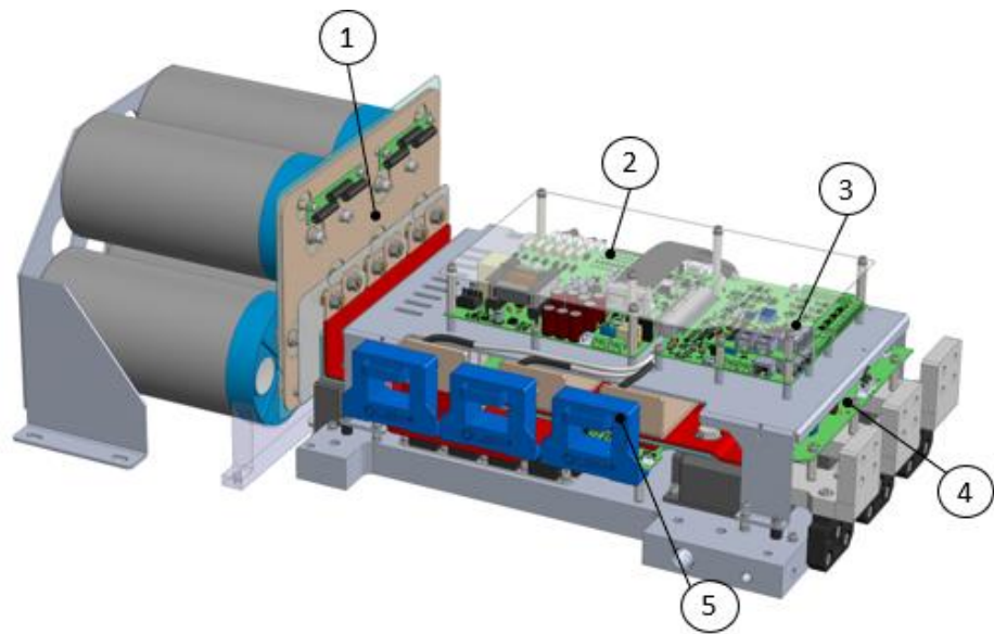
Abb.° 31 - Austauschbare Teile des VFD hervorgehoben
