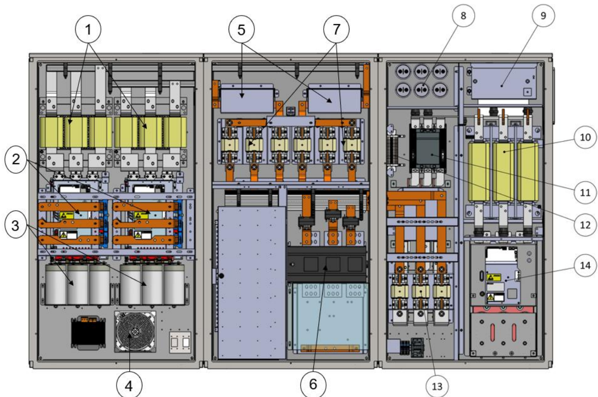
Abb.° 30 - Elemente der Schalttafel des VFD mit aktivem Filter
