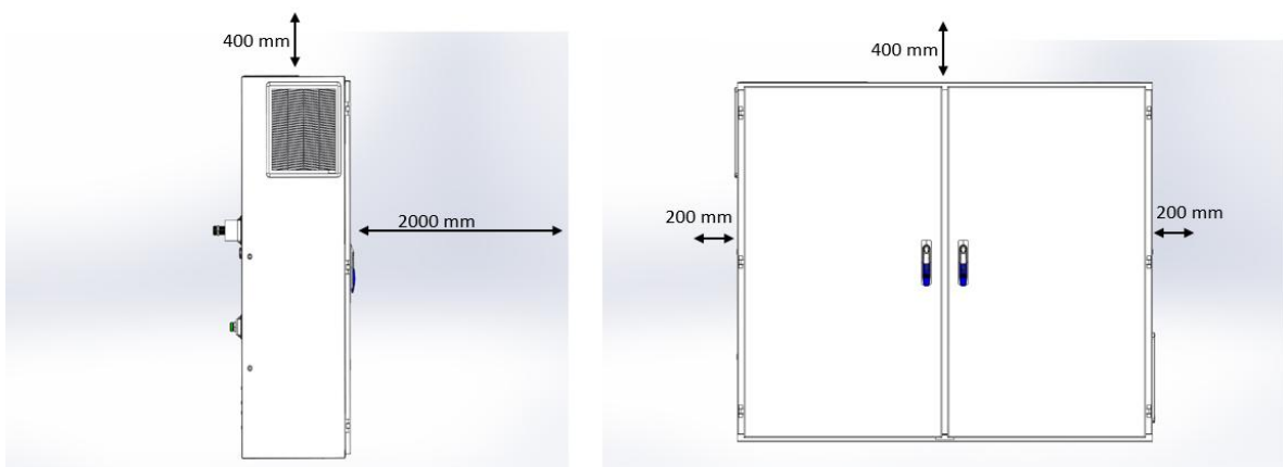
Abb.° 18 - Mindestabstände für VFD
