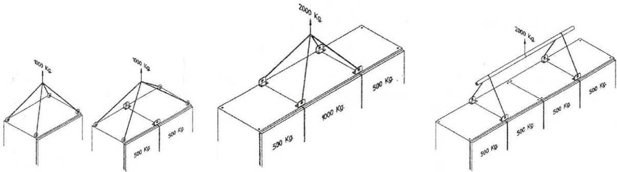
Abb.° 17 - Anheben des VFD
