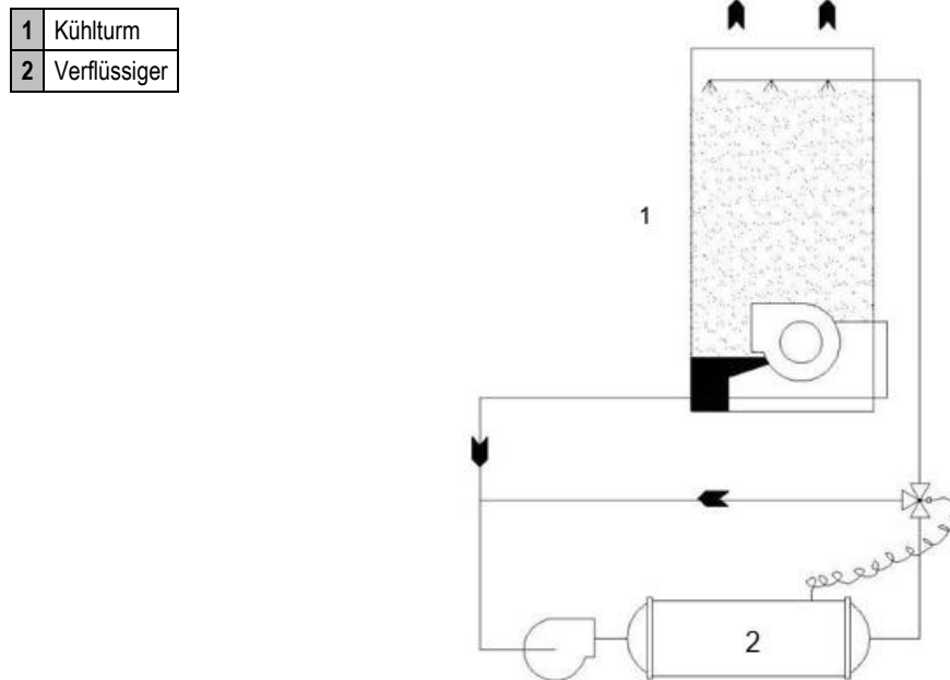
Abb.° 7 - Verflüssiger-Steuerschema mit Kühlturm
