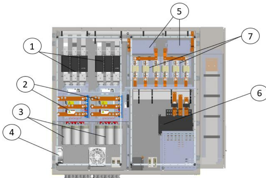
Abb.° 25 - Teile der Inverter-Schalttafel (Dual)
