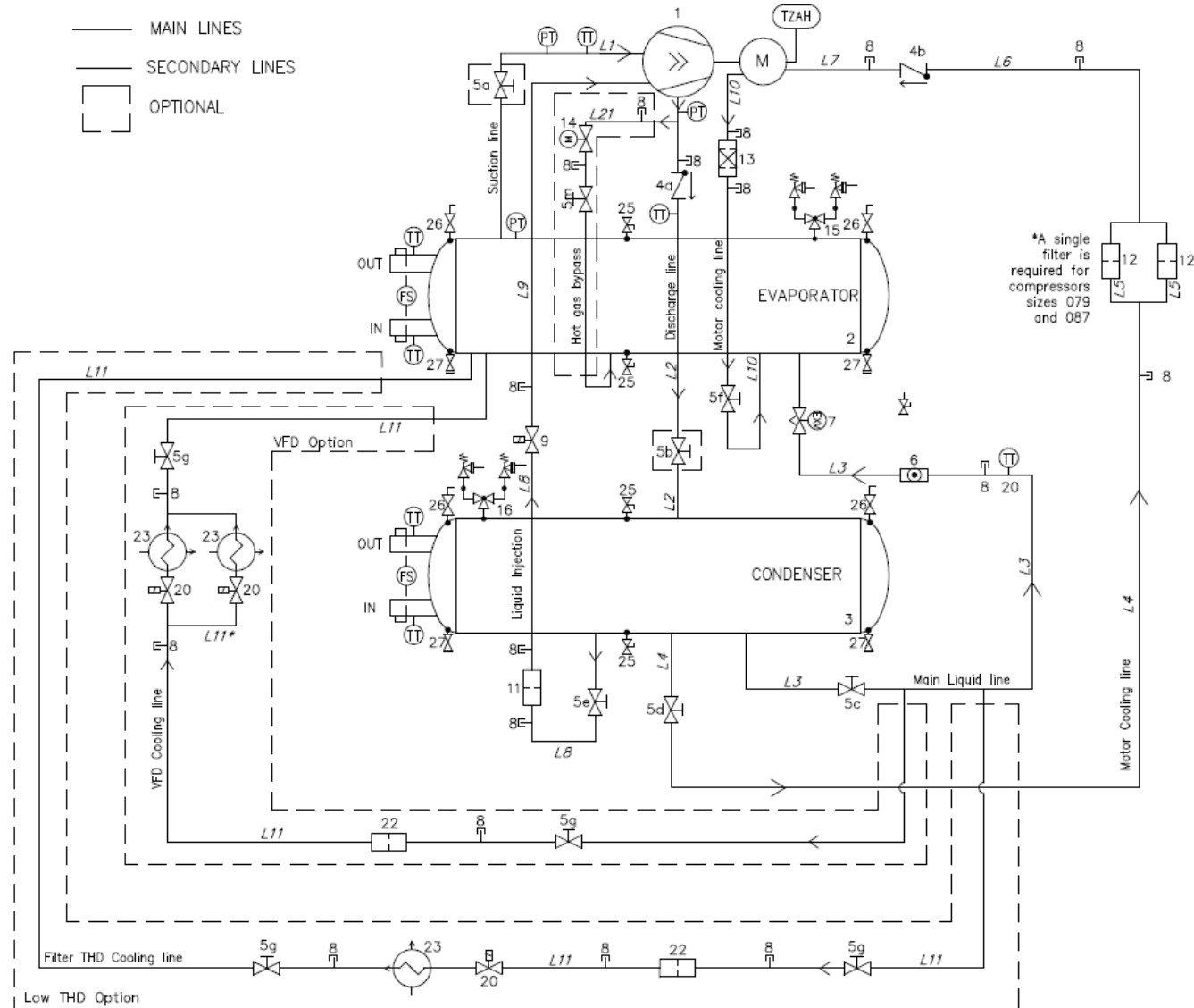
Darstellung von Wasserzu- und -ablauf ist als Beispiel zu verstehen. Die genauen Maße für die Wasseranschlüsse sind den Maßzeichnungen der Maschine zu entnehmen.
