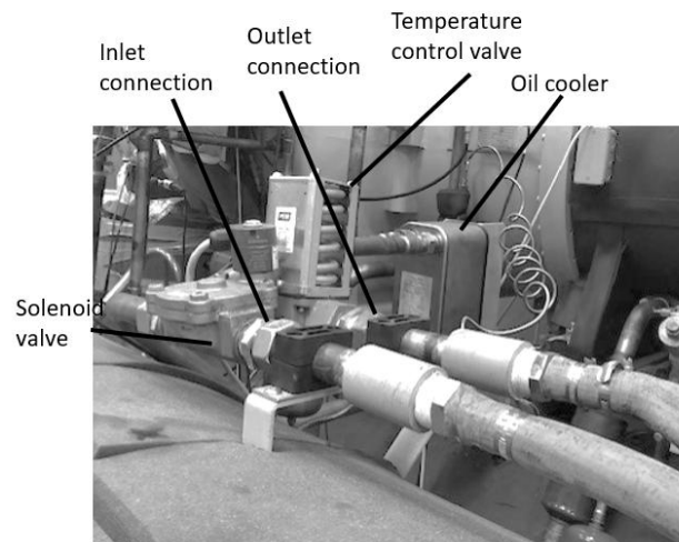
10. ábra- DWSC, az olajhűtés csatlakozásai
