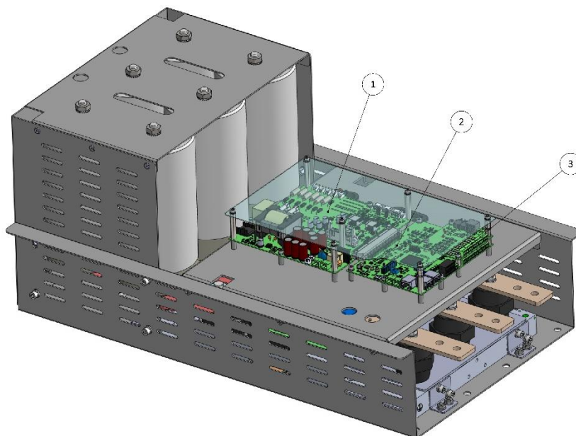
32. ábra - Az aktív szűrő cserélhető alkatrészei kiemelve
