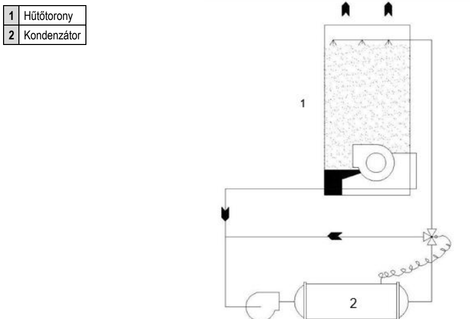
6. ábra - Kondenzátor vezérlési séma hűtőtoronnyal
