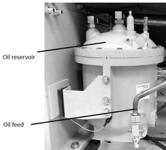
10. ábra- DWSC, az olajhűtés csatlakozásai
