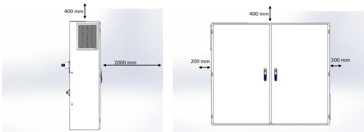
18.ábra - Minimálisan szükséges szabad hely a VFD karbantartásához
