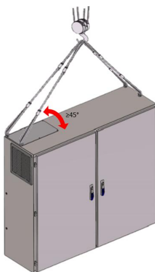
16.ábra - Megfelelő szög az emeléshez
