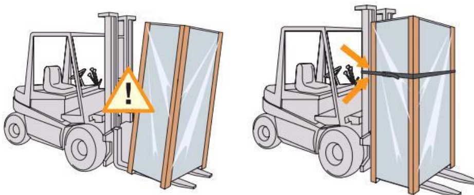
16.ábra - Megfelelő szög az emeléshez
