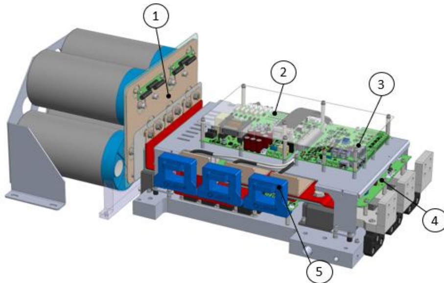
26. ábra - VFD cserélhető alkatrészei kiemelve
