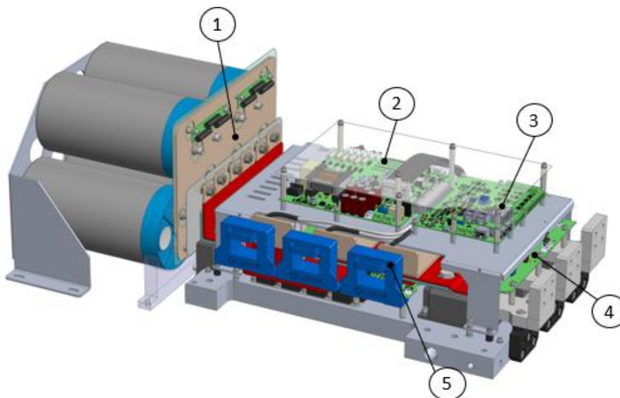
31. ábra - VFD cserélhető alkatrészei kiemelve
