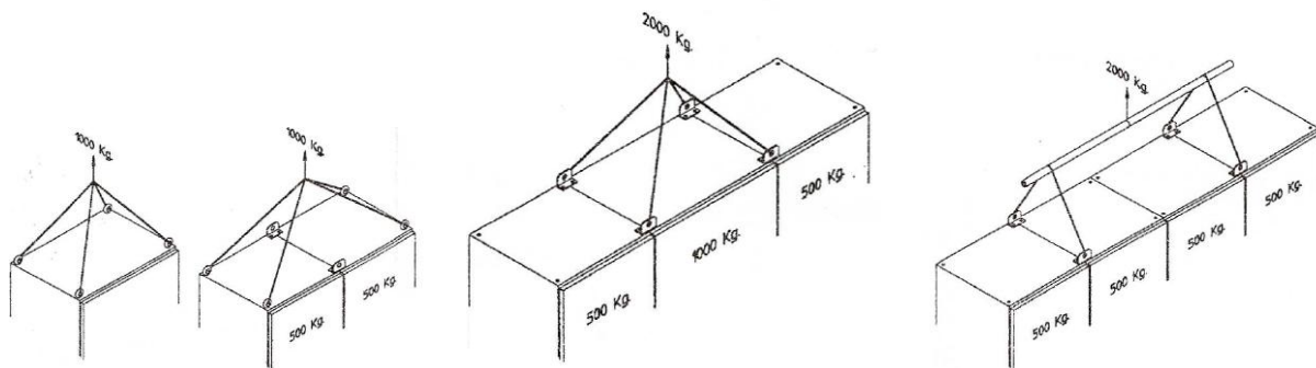
17.ábra - A VFD felemelése
