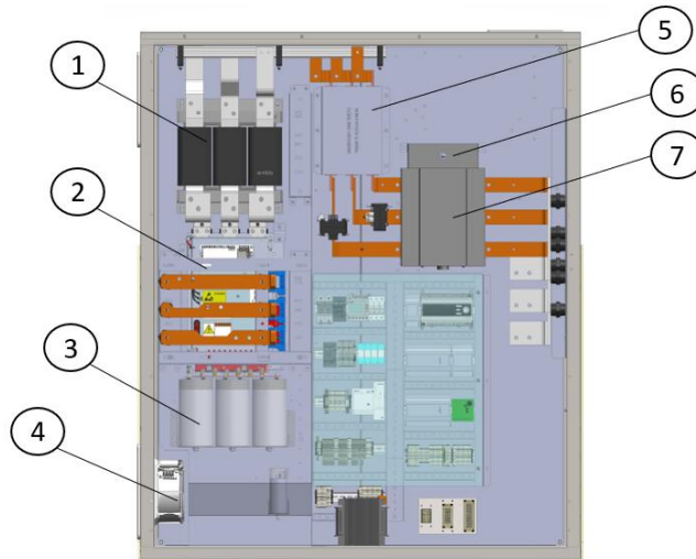
Afb. 26 - Onderdelen paneel omvormer (dual)
