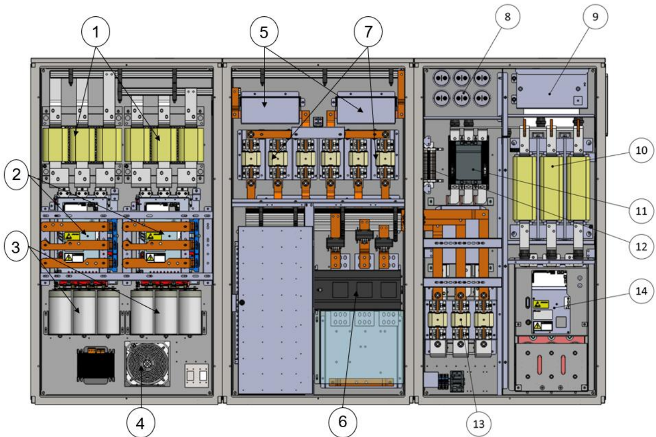
Afb. 31 - Onderdelen paneel van de VFD met actief filter
