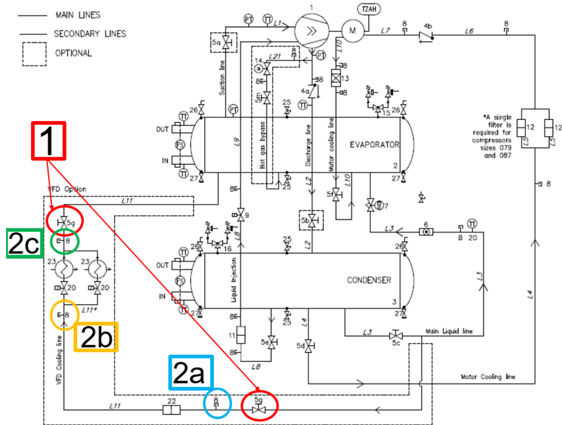
Afb. 28 - P&ID-schema van de unit met detail koelleiding omvormer
