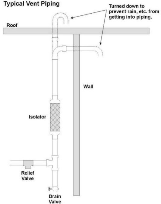
Afb. 12 - Typische ontluuchtingspijpen
