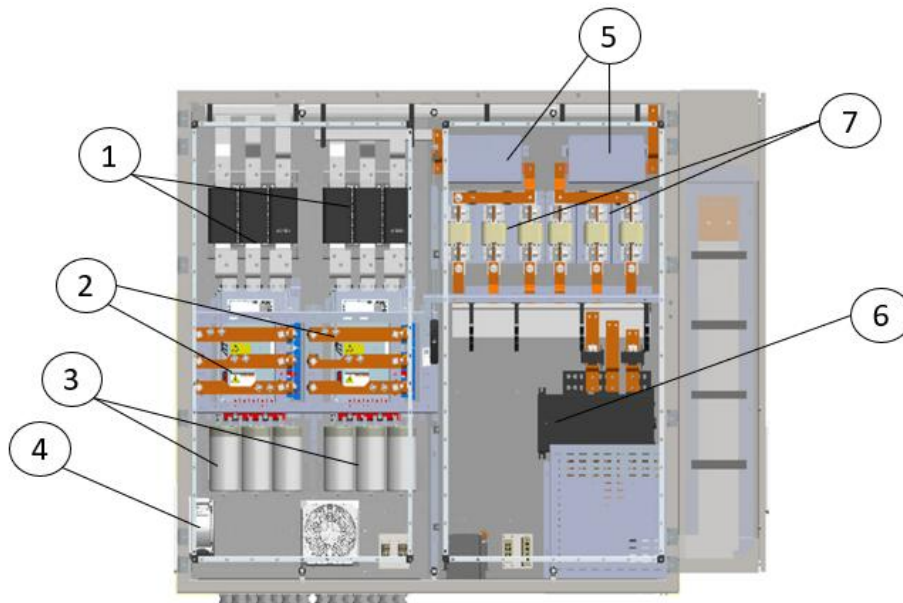
Afb. 26 - Onderdelen paneel omvormer (dual)
