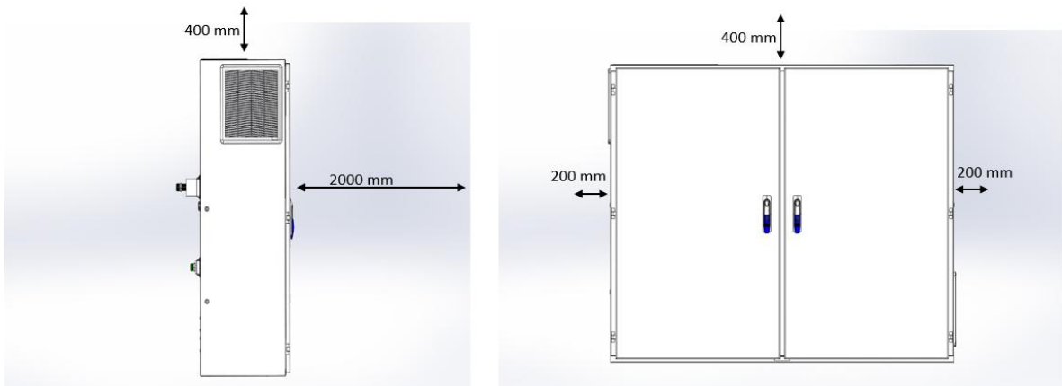
Afb. 19 - Minimaal vereiste ruimte voor VFD
