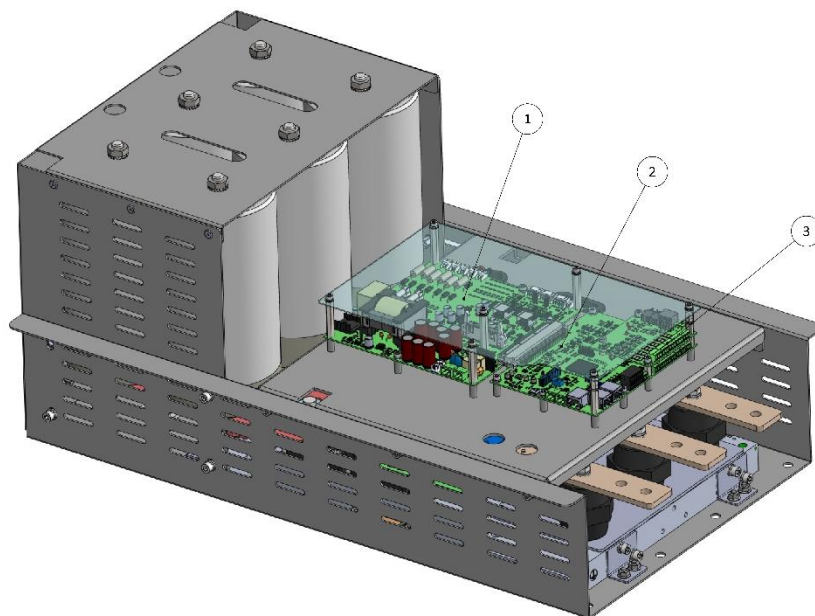
Afb. 33 - Gemarkerde reserveonderdelen actief filter
