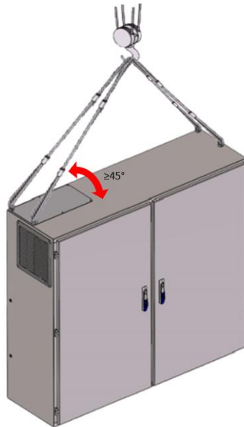
Afb. 17 - Na te leven hoek voor hefwerkzaamheden
