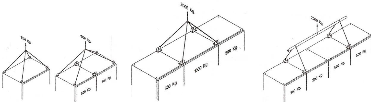
Afb. 18- De VFD heffen
