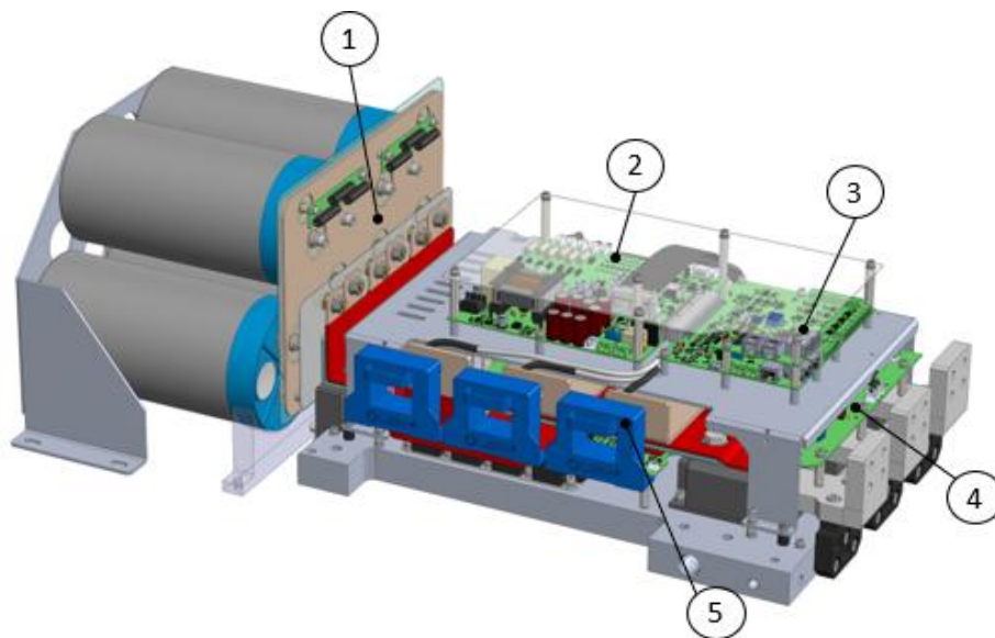
Afb. 32 - Gemarkerde reserveonderdelen VFD
