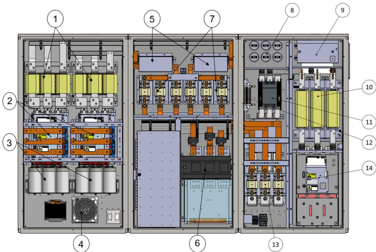
Рис. ° 31. Компоненты панели ЧРП с активным фильтром
