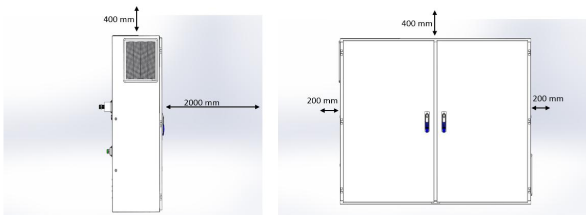
Рис. ° 19 Требования к расстоянию в свету для ЧРП
