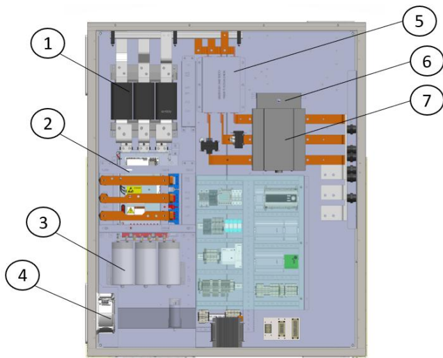
Рис. ° 26. Компоненты (сдвоенной) панели инвертора
