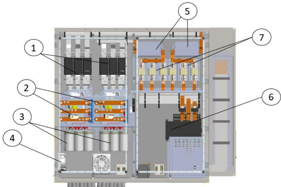
Рис. ° 26. Компоненты (сдвоенной) панели инвертора
