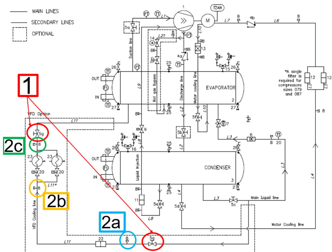
Рис. ° 28 . Схема трубопроводов и КИП агрегата с выносным элементом линии охлаждения инвертора
