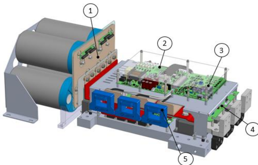
Рис. ° 27 . Выделены сменные детали ЧРП
