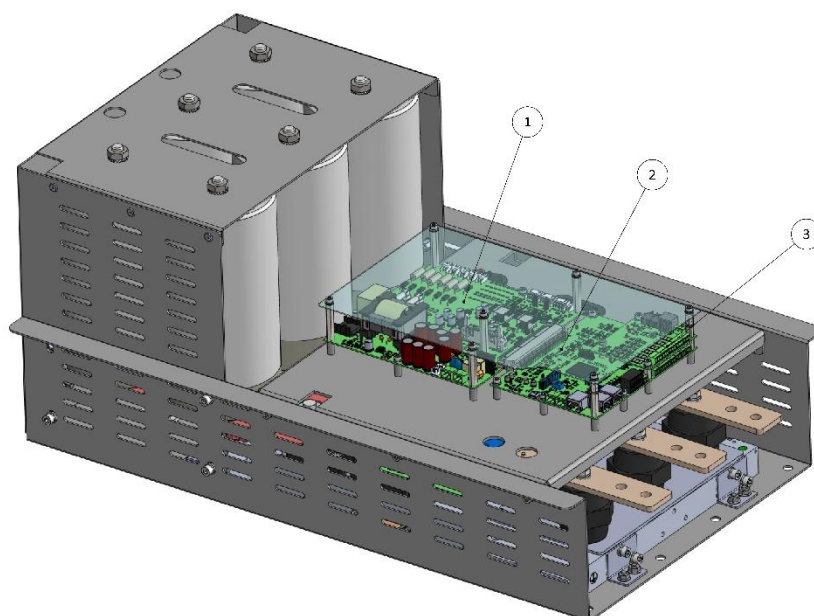
Рис. ° 33. Выделены сменные детали активного фильтра
