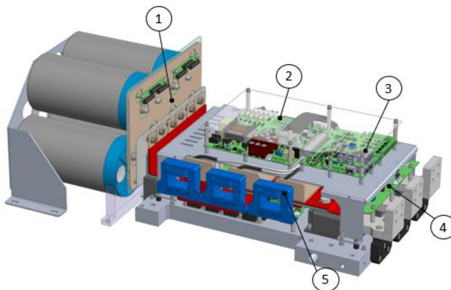
Рис. ° 32. Выделены сменные детали ЧРП
