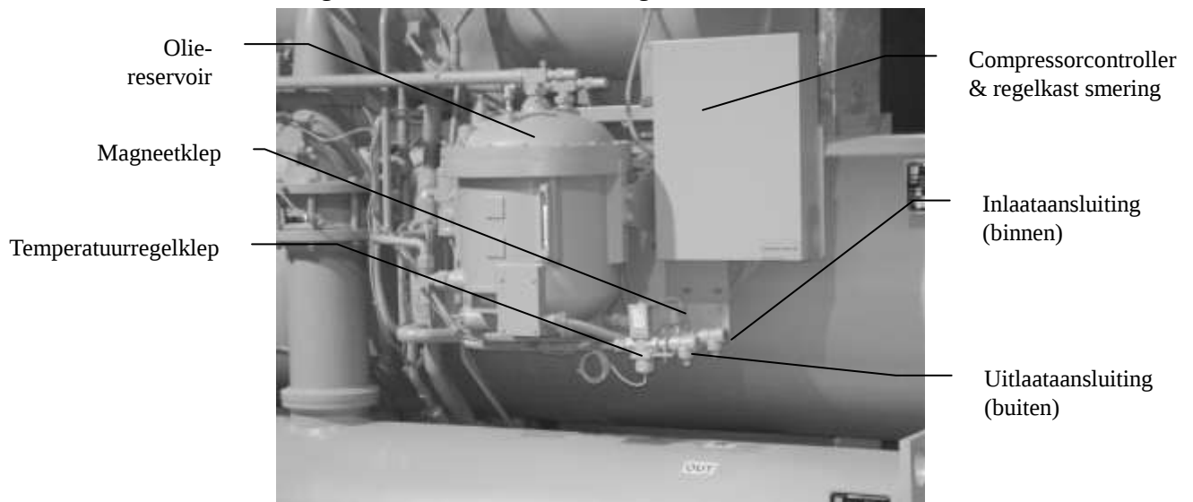
Afbeelding 11, Oliekoeleraansluitingen, DWSC/DHSC-units
