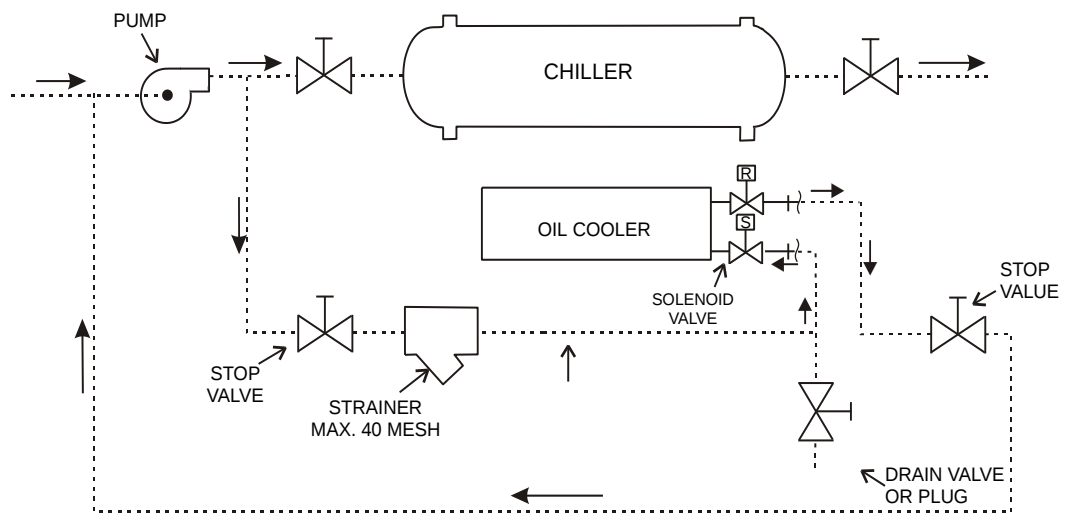
Afbeelding 9, Oliekoelerleiding over pomp voor gekoeld water
