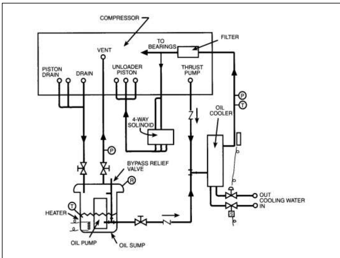
Afbeelding 24, Typisch oliestromingsschema
