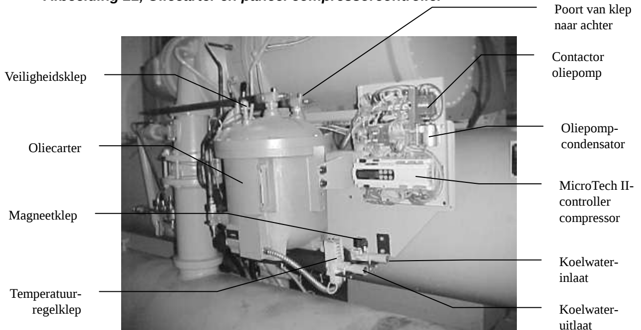
Afbeelding 21, Oliecarter en paneel compressorcontroller
