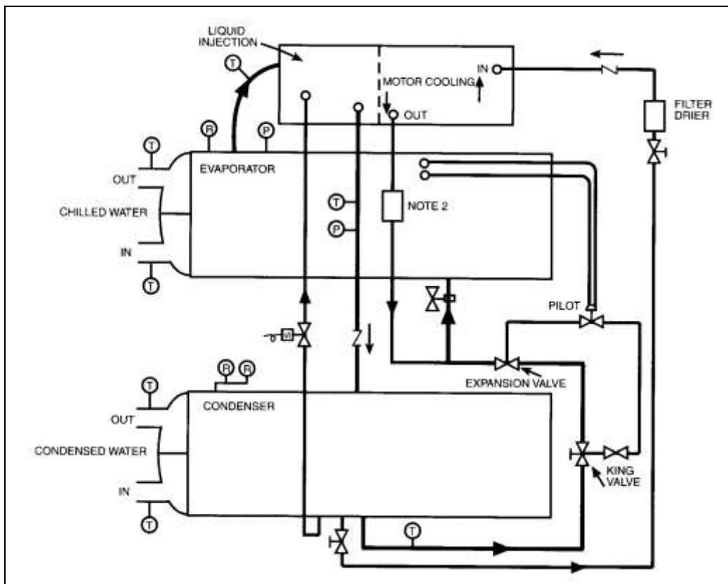
Afbeelding 25. Schema typische koelmiddelstroming
