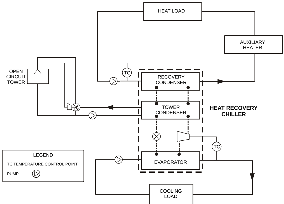
Afbeelding 7, Schema warmteterugwinning
