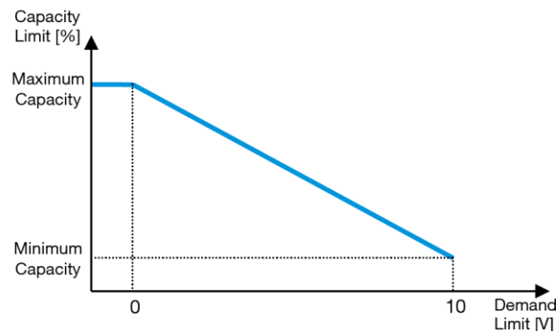
Diagramm 2 – Bedarfsgrenze[V] vs. Kapazitätsgrenze[%]
