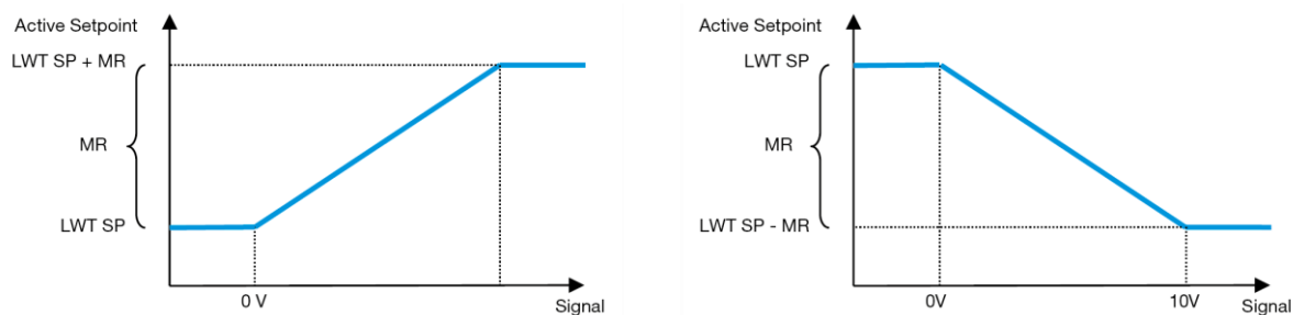
Grafico 4 – Segnale esterno 0–10 V vs setpoint attivo – modalità Raffreddamento (sinistra) / modalità Riscaldamento (destra).
