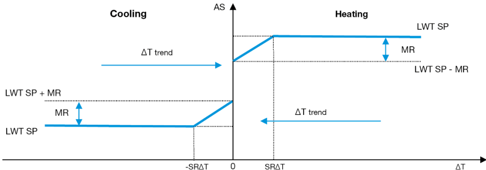
Grafico 5 – \Delta T evaporatore vs Setpoint Attivo – modalità Raffreddamento (sinistra) / modalità Riscaldamento (destra)
