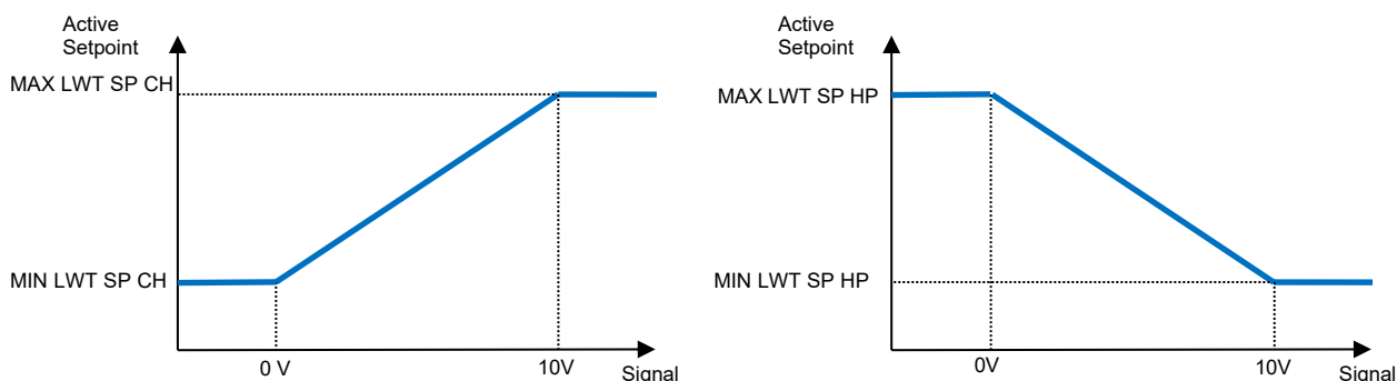
Grafico 6 – Segnale esterno 0–10 V vs Setpoint LWT sovrascritto in modalità Raffreddamento (sinistra) e modalità Riscaldamento (destra)
