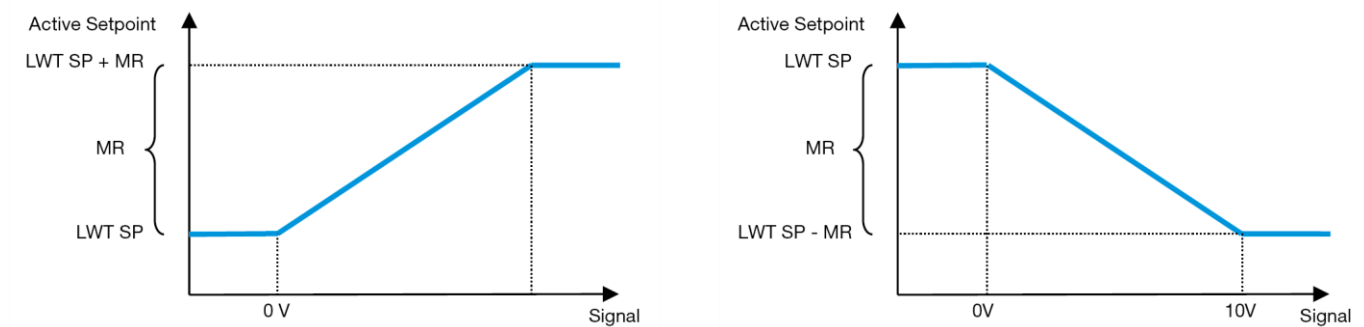
Graafik 2 – Välissignaali 0-10 V vs Aktiivne Seadepunkt - Jahutusrežiim(vasakul)/ Kuumenemisrežiim(paremal)
