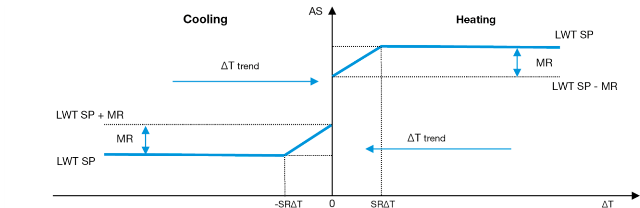
Graafik 3– Aurusti \Delta T vs Aktiivne Seadepunkt - Jahutusrežiim(vasakul)/ Kuumenemisrežiim(paremal)
