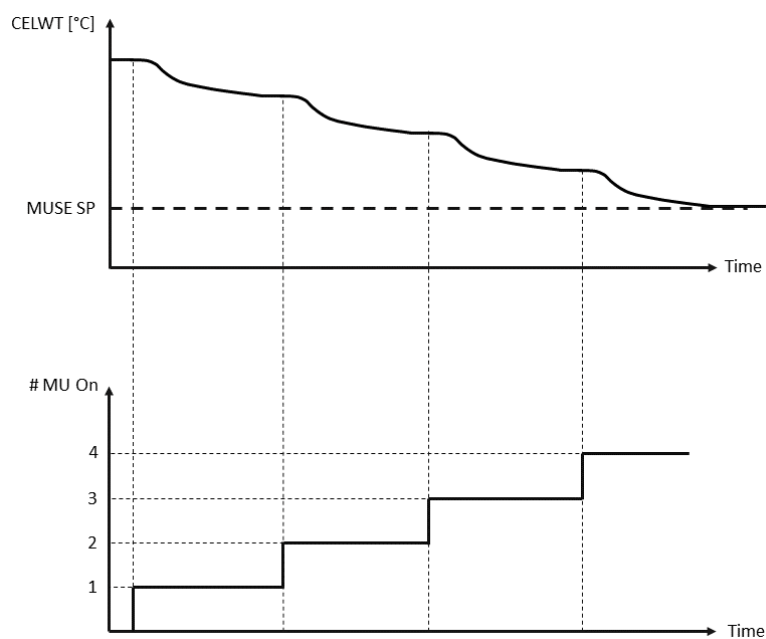
Graafik 4 - Moodulseadete käivitusjärjestus - Jahutusrežiim
