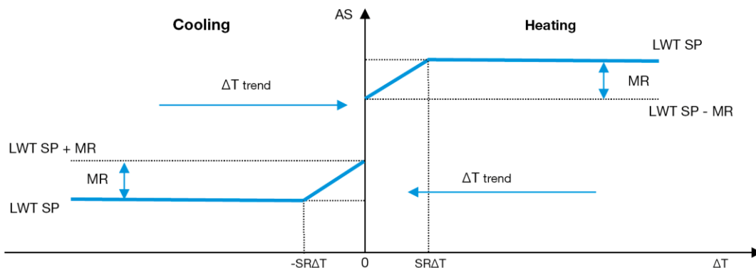
Kuvaaja 3– Evap \Delta T vs. aktiivinen asetusarvo - Jäähdystystila (vasen) / Lämmitystila (oikea)
