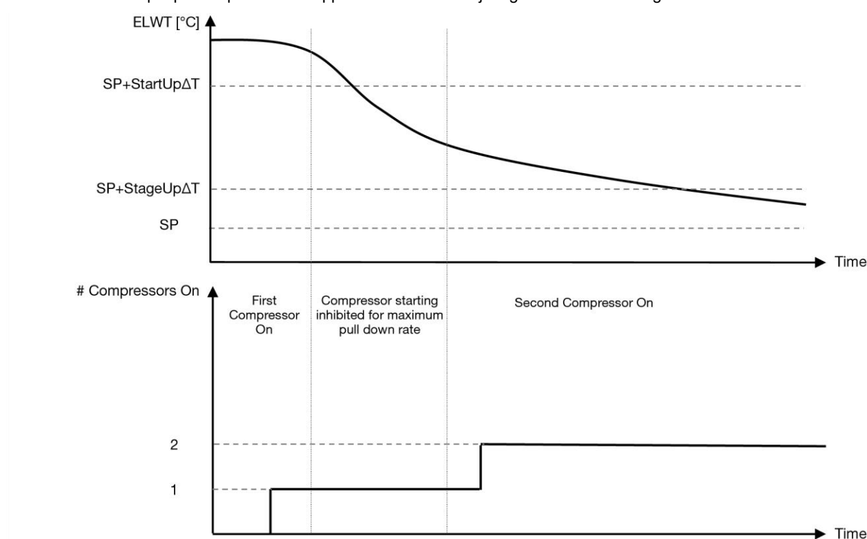
Graf 1 – Kompressorer oppstartssekvens - Kjølemodus
