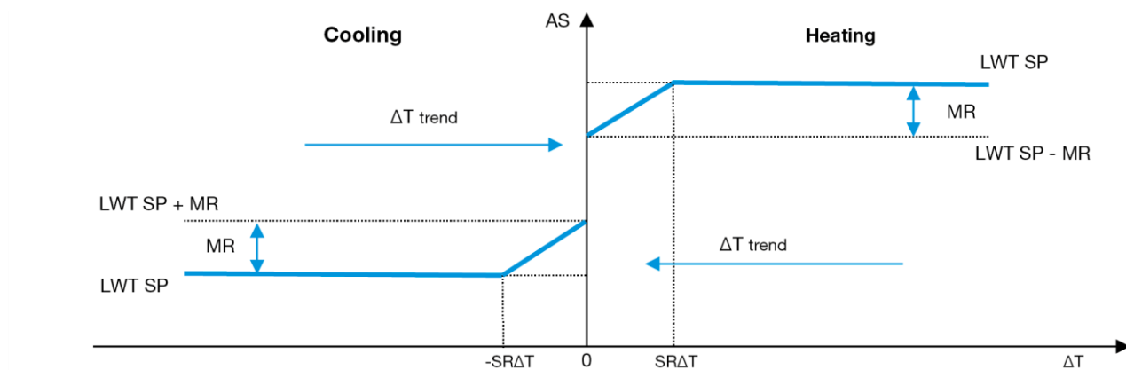
Graf 3– EvapT vs Aktivt settpunkt - Kjølemodus(venstre)/ Oppvarmingsmodus(høyre)
