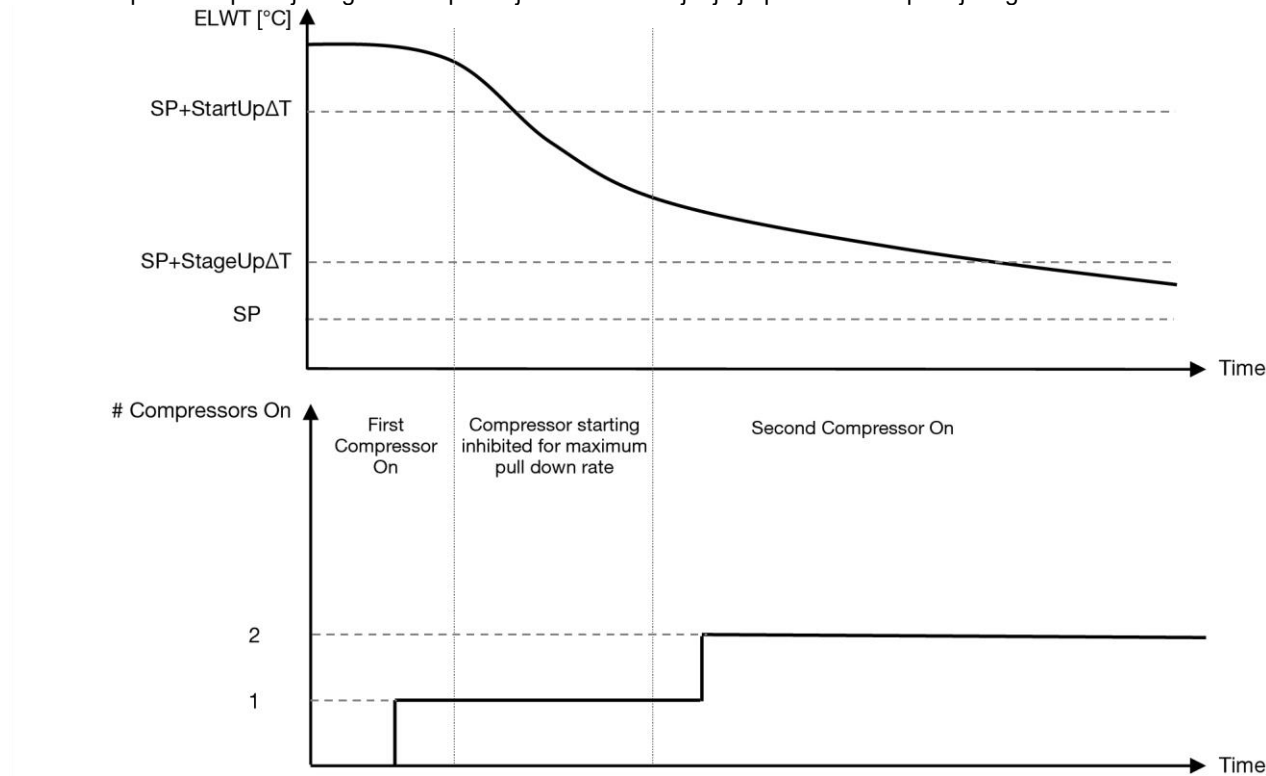
Diagram1 – Zaporedje zagona kompresorjev - Cool mode
