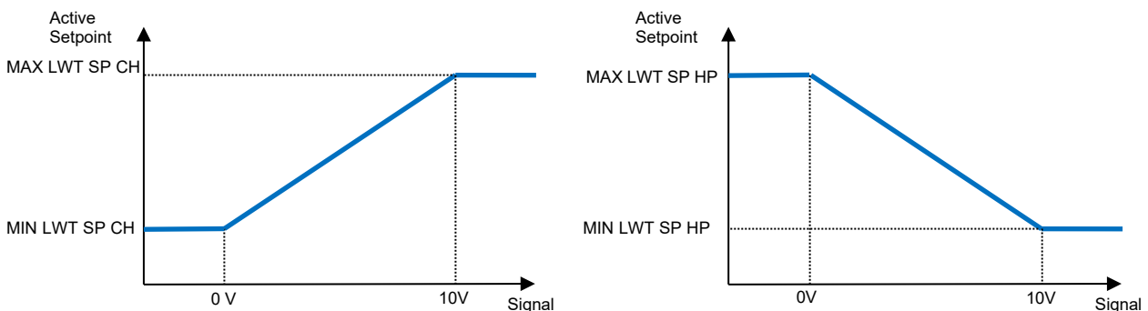
Graf 6 – 0–10 V externí signál vs cíl Lwt přepsán v režimu chlazení (vlevo) a režimu vytápění (vpravo)
