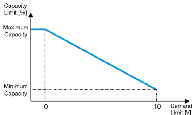
Diagramm 2 – Bedarfsbegrenzung [V] gegenüber Kapazitätsgrenze [%]
