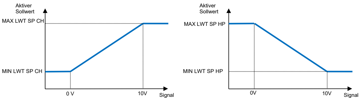
Diagramm 6 – 0-10V Externes Signal vs. Lwt-Ziel überschrieben im Kühlmodus (links) und Heizmodus (rechts)
