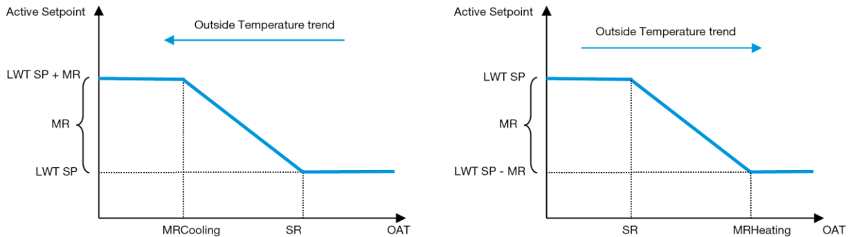
Diagramm 3 – Außentemperatur gegenüber aktivem Sollwert – Kühlmodus (links)/Heizmodus (rechts)
