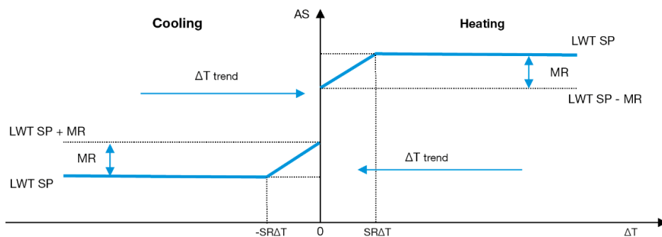
Γράφημα 5 – Έναρ ΔT (Διαφορά θερμοκρασίας για εξατμιστή) και Ενεργό Σημείο Ορισμού - Λειτουργία Ψύξης (αριστερά) / Λειτουργία Θέρμανσης (δεξιά)
