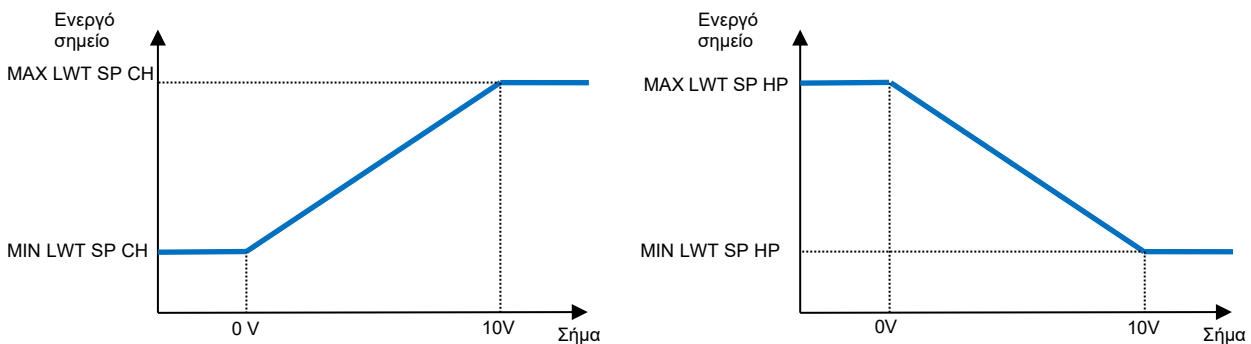
Γράφημα 6 – 0-10V Εξωτερικό Σήμα εναντίον του Στόχου που αντικαθίσταται στη Λειτουργία Ψύξης (Αριστερά) και τη Λειτουργία Θέρμανσης (Δεξιά)
