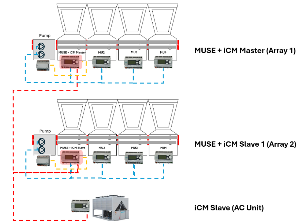
Schéma de configuration MUSE + iCM
