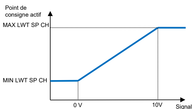
Graphique 6 – Signal externe 0-10 V par rapport à la cible LWT écrasée en mode refroidissement (gauche) et en mode chauffage (droite)
