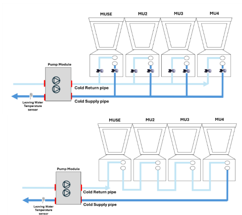
Schematy konfiguracji MUSE równoległej i szeregowej
