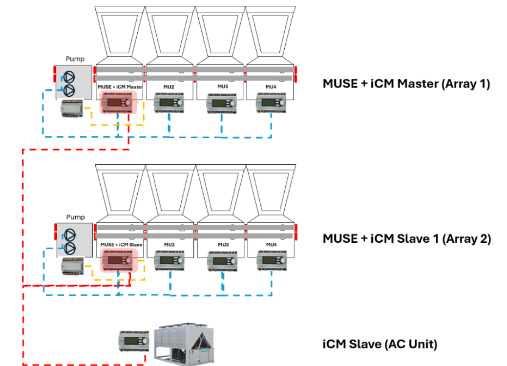
Esquema de configuración de MUSE + iCM
