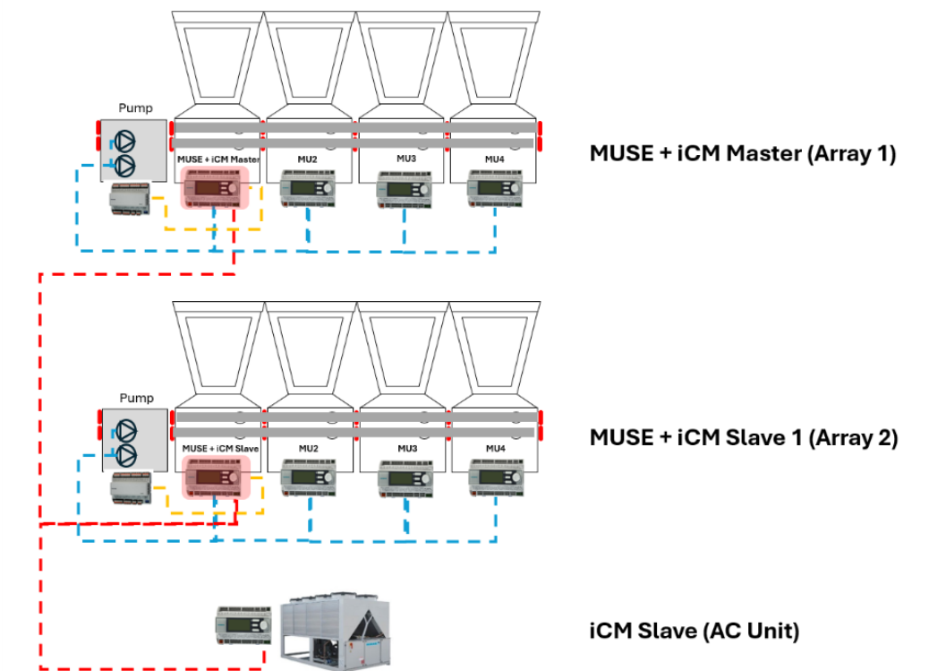
Schéma de configuration MUSE + iCM
