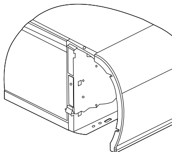
Ventilconvettore senza zoccolo
