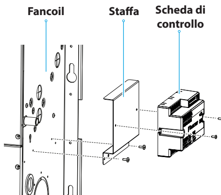
Schema di montaggio
